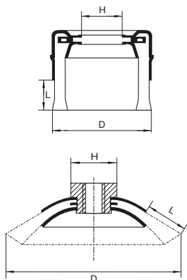
Dimensiuni Perie tip oală și conică
