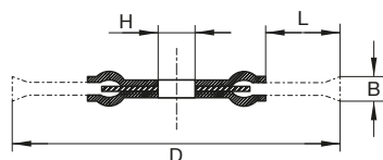
Dimensiuni Perii rotunde
