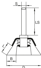
Dimensiuni Perii oală montate pe ax
