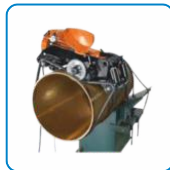
Mașini de șanfrenat pentru muchii sau pentru țevă
