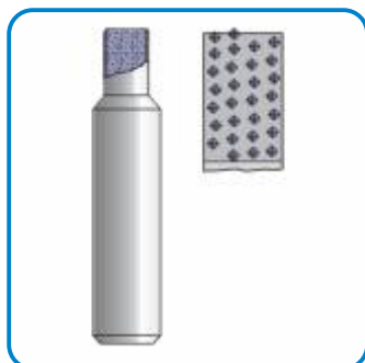
Corpuri cu plăci cu diamante multigranulă multilaterale, pentru rectificare
